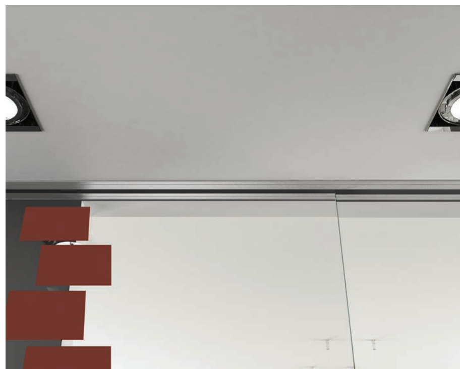
DETTAGLIO SISTEMA CON BINARIO INVISIBILE SCM-7000 PER MONTAGGIO INTEGRATO NEL SOFFITTO/CONTROSOFFITTO DETAIL OF SCM-7000 SYSTEM WITH CONCEALED RAIL FOR INSTALLATION SET INTO CEILING / SUSPENDED CEILING
